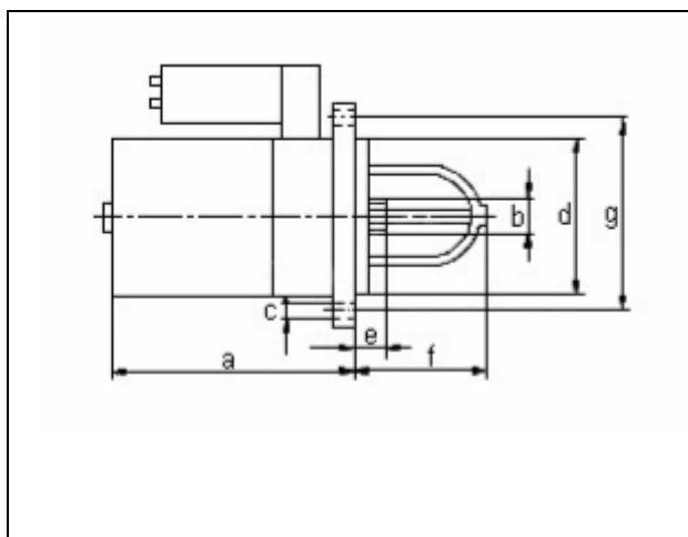
Моторы : VA + F2 + FE
