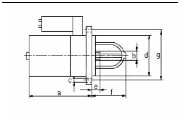
Мотор : MAZDA VA + FE
