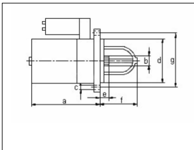
Моторы : 2Z + 1DZ + 11Z
