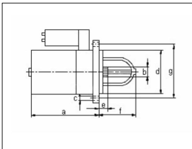
Моторы : SD22 + SD25
